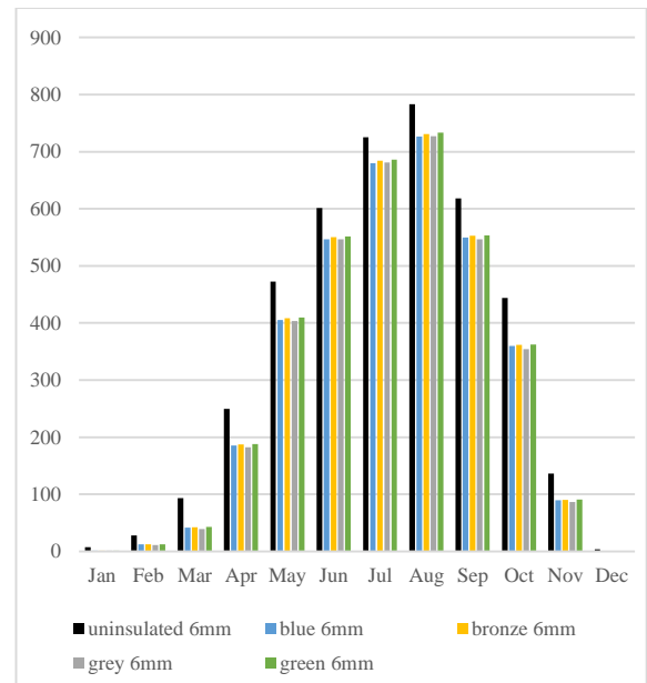
نمودار ۲: مقایسه‌ی بار سرمایشی محاسبه‌شده در شیشه‌های یک‌لایه (Kwh)
