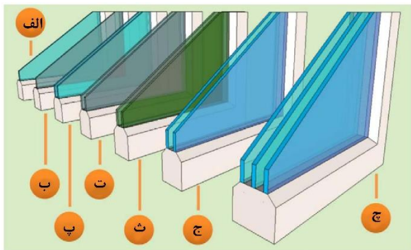
شکل ۲: الف) پنجره‌ی تک‌لایه با شیشه‌ی معمولی؛ ب) پنجره‌ی تک‌لایه با شیشه‌ی خاکستری؛ پ) پنجره‌ی دولایه با شیشه‌ی معمولی؛ ت) پنجره‌ی دولایه با شیشه‌ی رنگی؛ ث) پنجره‌ی دولایه با شیشه‌ی سبز؛ ج) پنجره‌ی دولایه‌ی کم‌گسیل؛ چ) پنجره‌ی سه‌لایه‌ی کم‌گسیل [۲۶].
