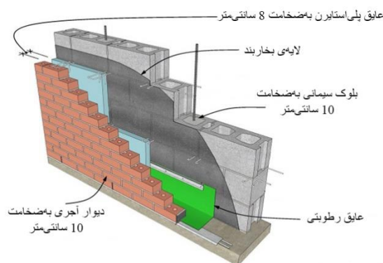
شکل ۴: جزئیات دیوار در نمونه‌های شبیه‌سازی شده
